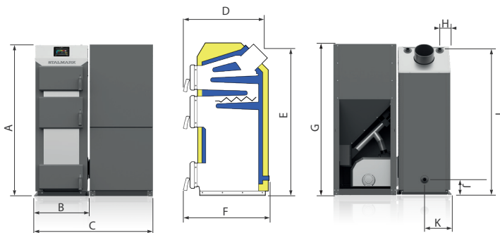
Wymiary - kotły typu PELLET TEXAS
